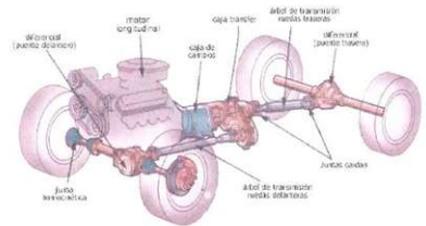
Esquema de transmisión para un vehículo de tracción a las 4 ruedas.
